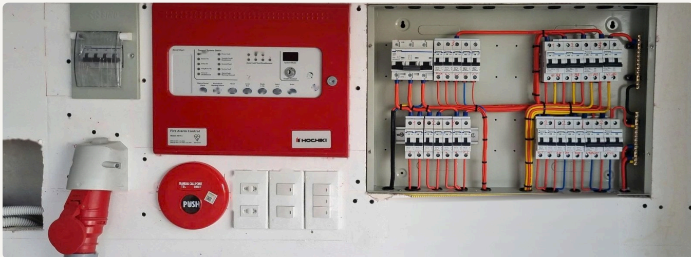
Vách kỹ thuật cửa hàng: tủ điện tổng chia nhánh có đánh số, tủ trung tâm báo cháy, nút ấn khẩn
